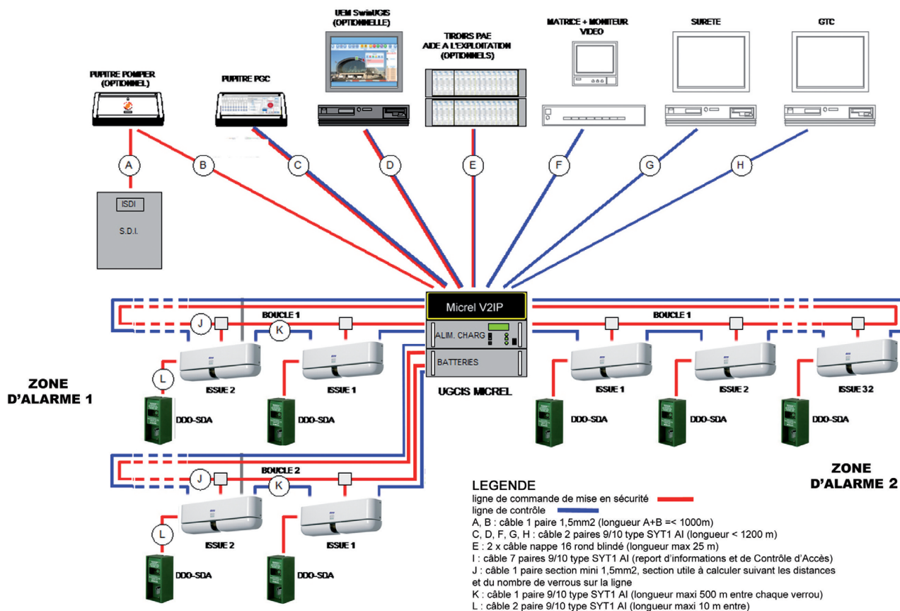
Synoptique d'installation
