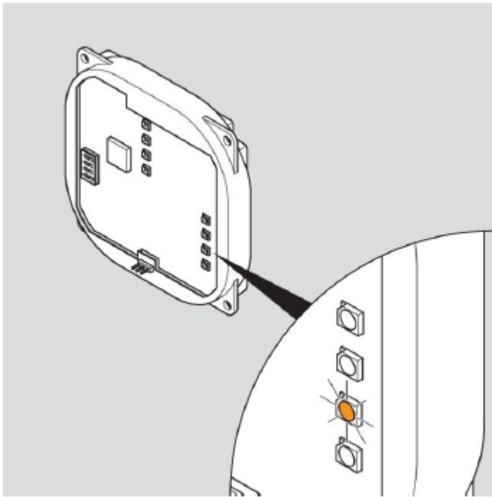
Prinzipdarstellung ENiQ/DOM Tapkey
