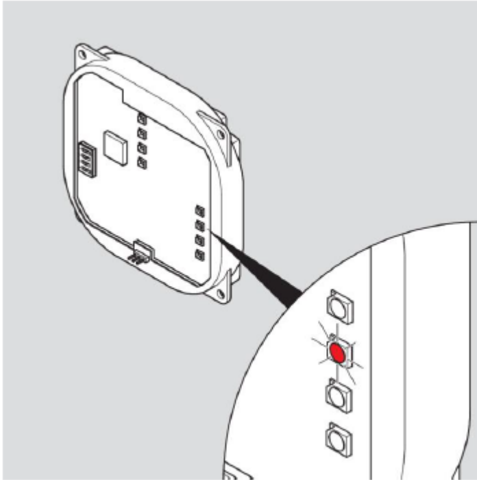
Prinzipdarstellung ENiQ
