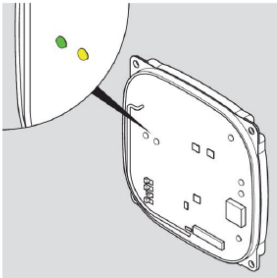
Prinzipdarstellung ELS
